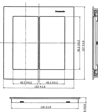
鋁合金 / 不鏽鋼蓋板 (2連用)
